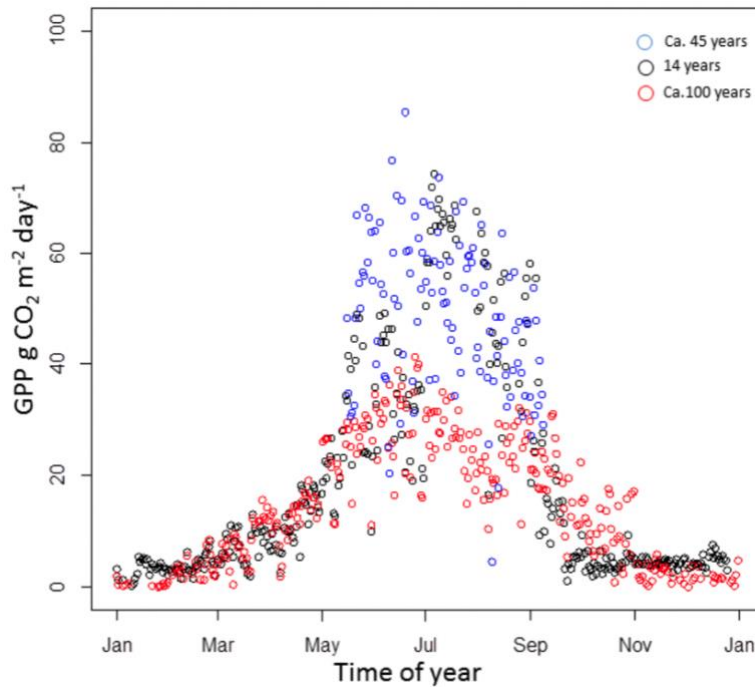
Fig 3. Dagligt utsläpp i medeltal för träd av olika åldrar
