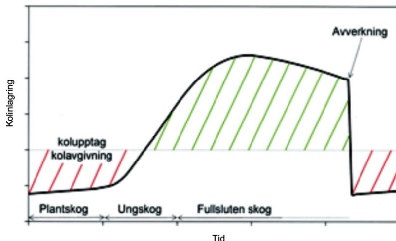
Fig 4. Det grönstreckade området indikerar att skogen tar upp mer koldioxid än den avger. I det röstreckade området är förhållandena de motsatta.
